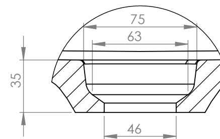
DETALLE L ESCALA 2 : 5
