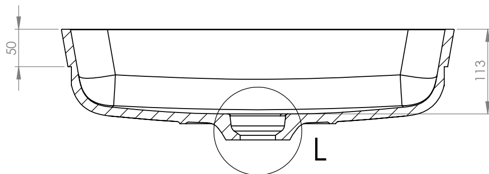
SECCIÓN K-K ESCALA 1 : 5
